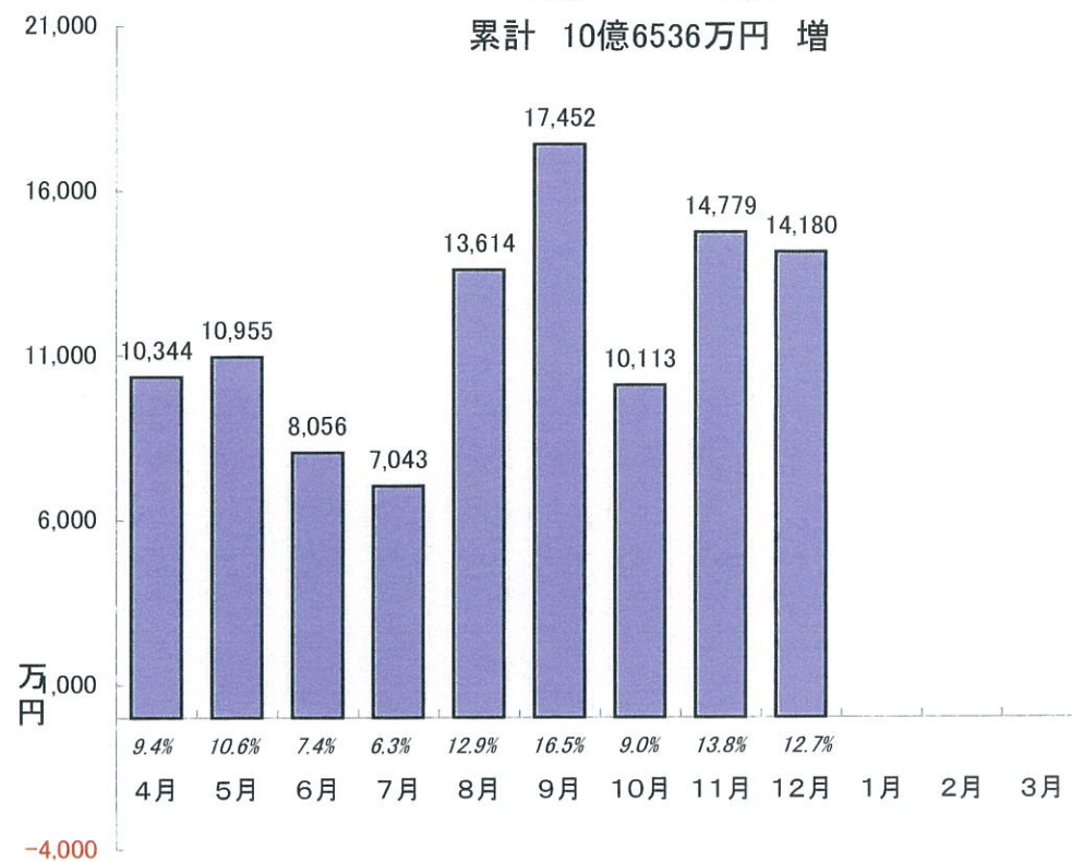
入院・外来 稼働額増減 前年同月比較 H21年度 : H22年度
