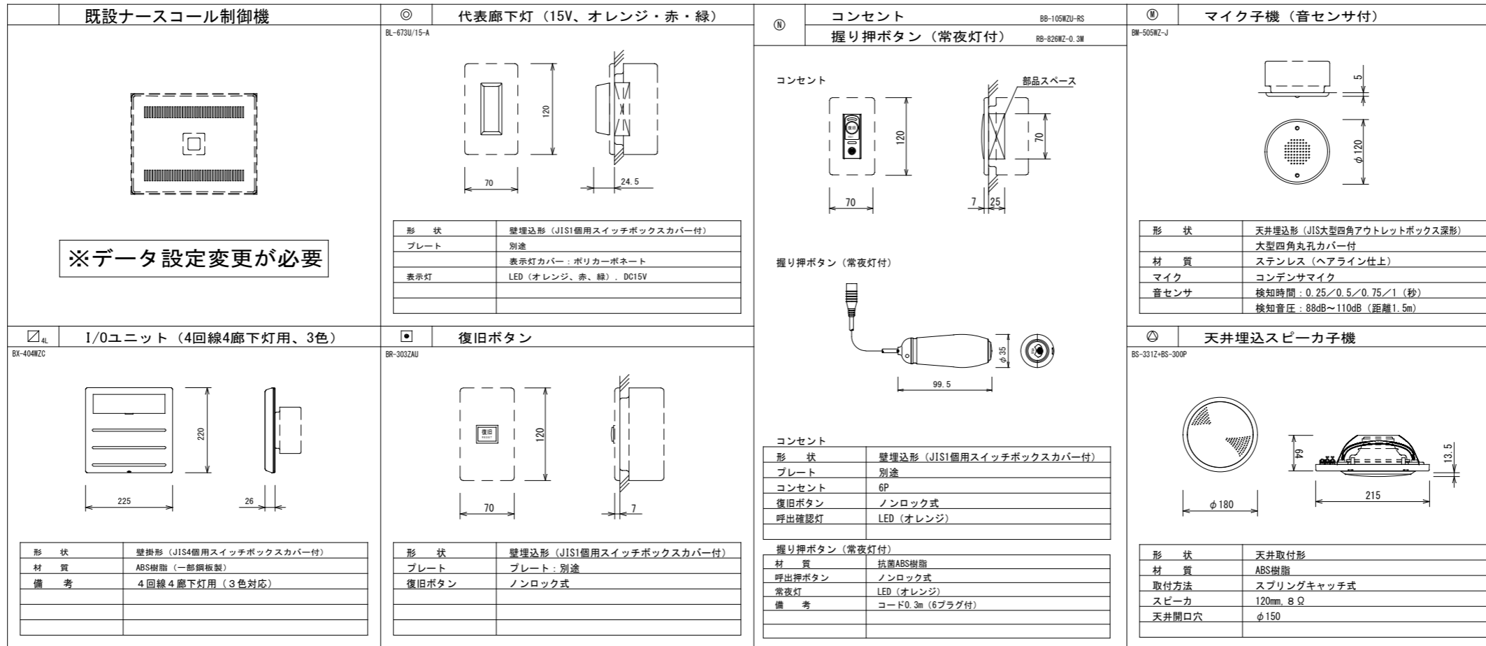
ナースコール設備 姿図
