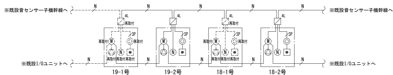
ナースコール設備 系統図
